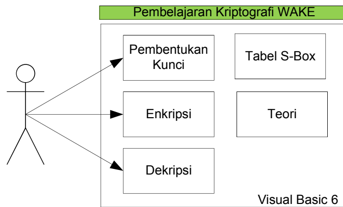
Gambar 1. Arsitektur Aplikasi
