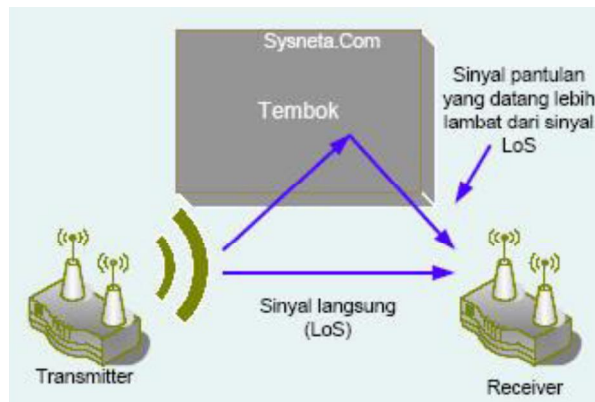
Gambar 2 Teknologi MIMO
