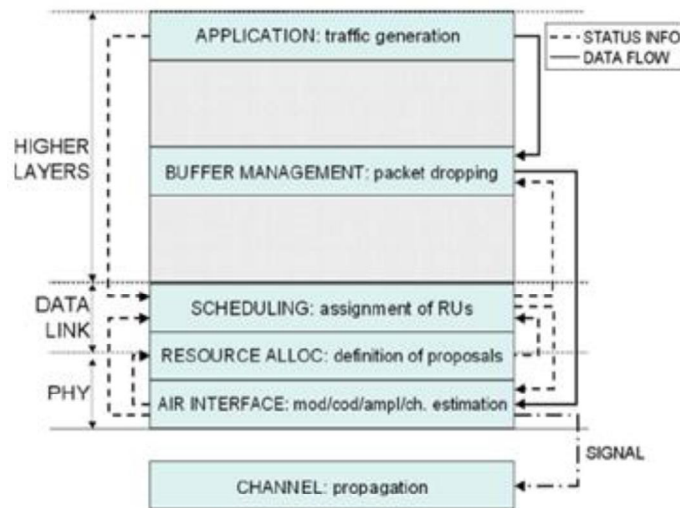
Gambar 3. Hubungan antar layer dan implementasinya
