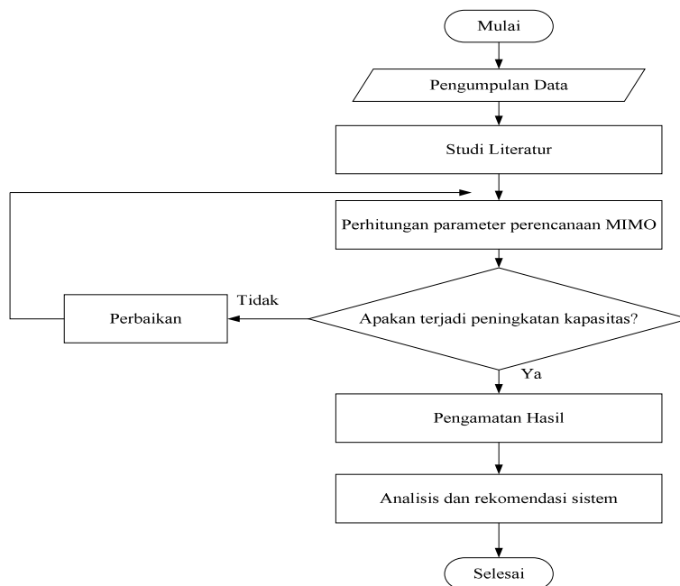
Gambar 4. Metodologi penelitian
